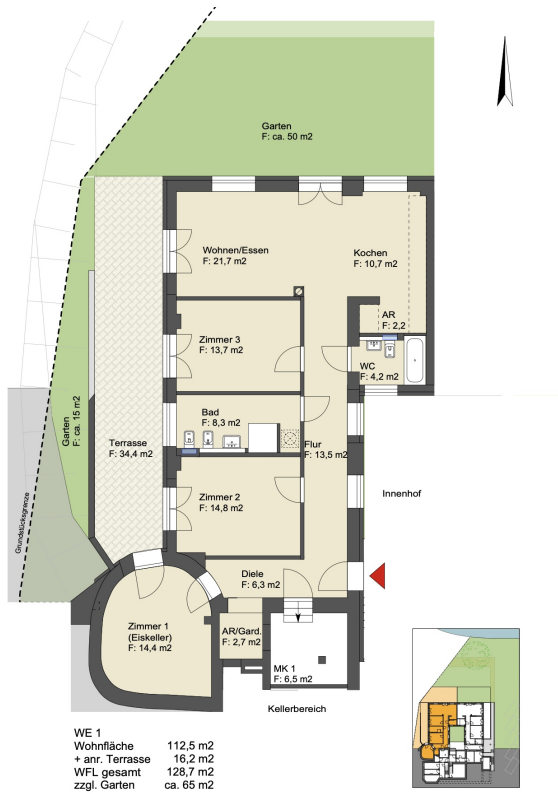
Grundriss
