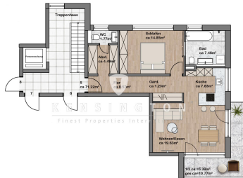
Wohnung Nr.5 Obergeschoss/ ca. 71.22m 2
