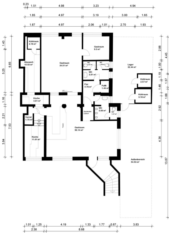
Grundriss
