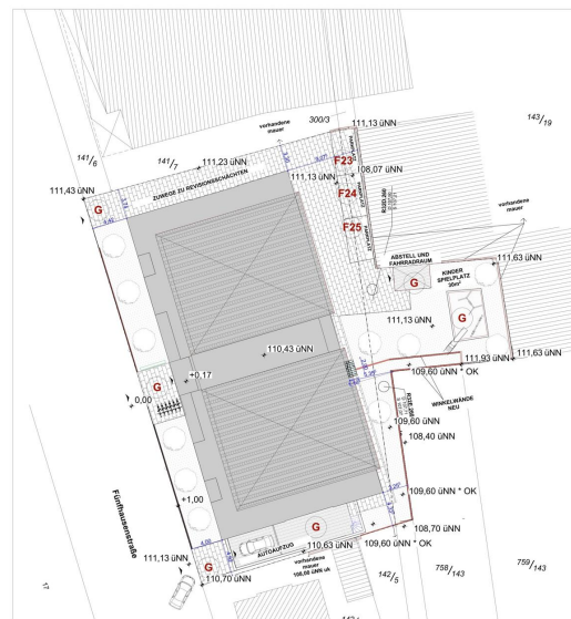
LAGEPLAN M=1:200
