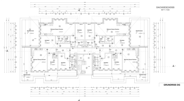
Grundriss_DG
