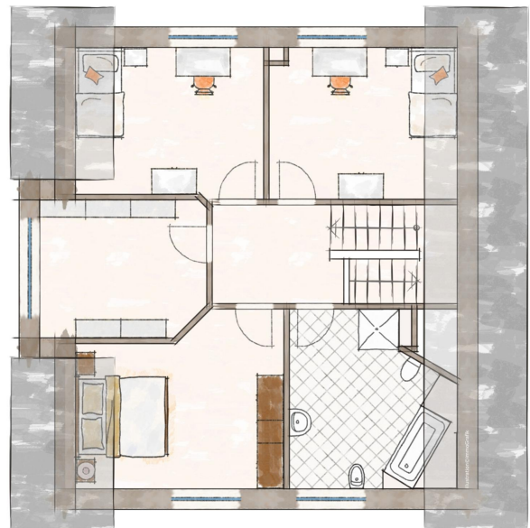
Obergeschoss
