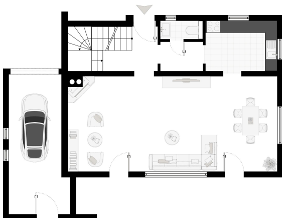
Grundriss EG
