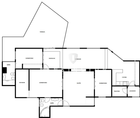
28 plano
