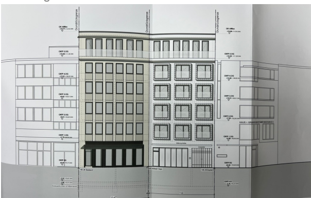
Planung Baulücke
