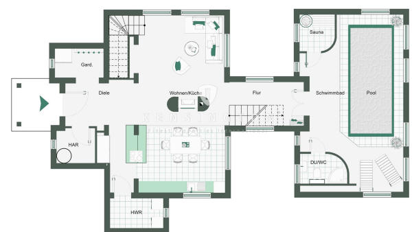
Grundriss Erdgeschoss
