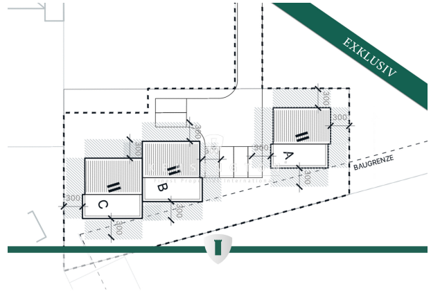
Skizze - Bauvorbescheid
