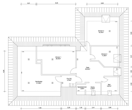
Dachgeschoss
