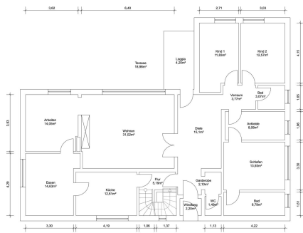
Erdgeschoss
