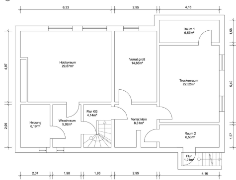
Kellergeschoss
