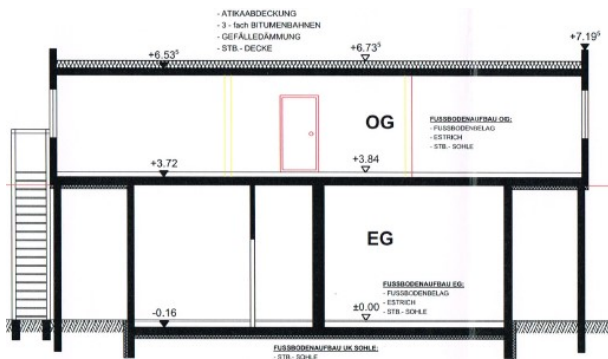
Schnitt
