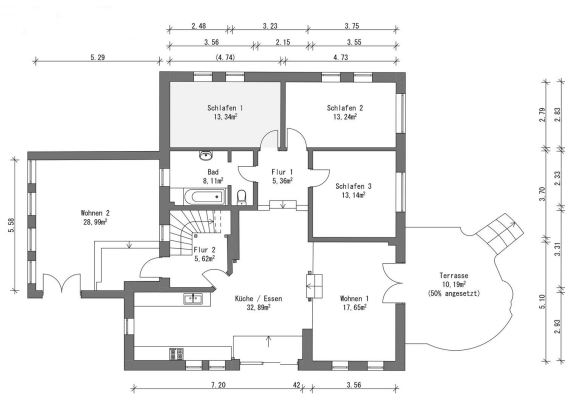
Erdgeschoss
