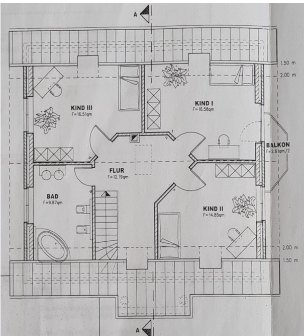
Grundriss_OG
