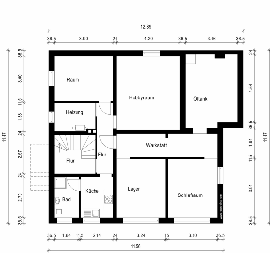
Grundriss_Keller
