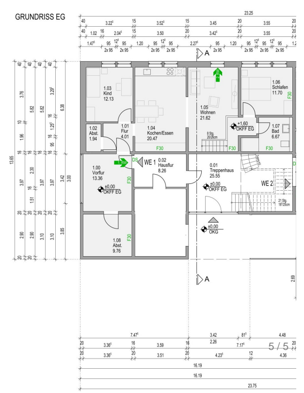
Grundriss
