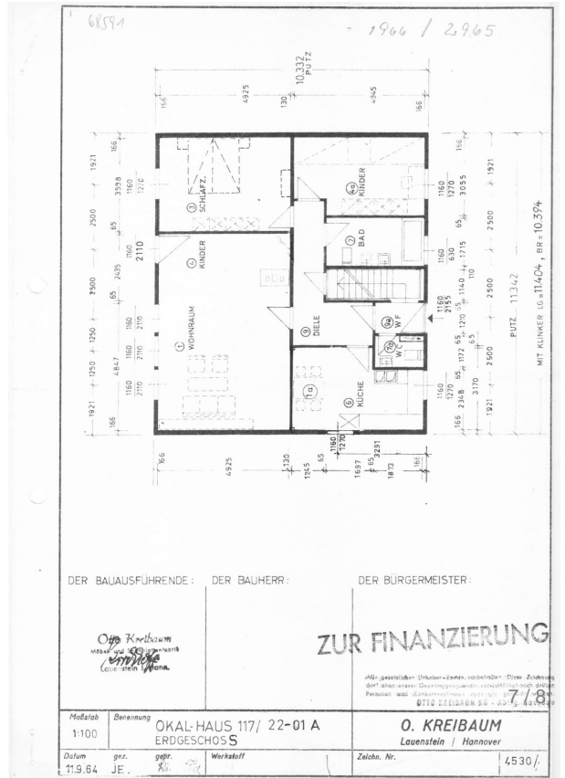
Grundriss_EG
