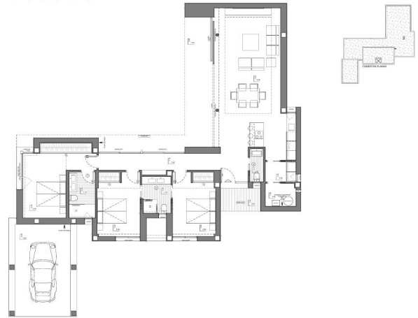
Grundriss AM033
