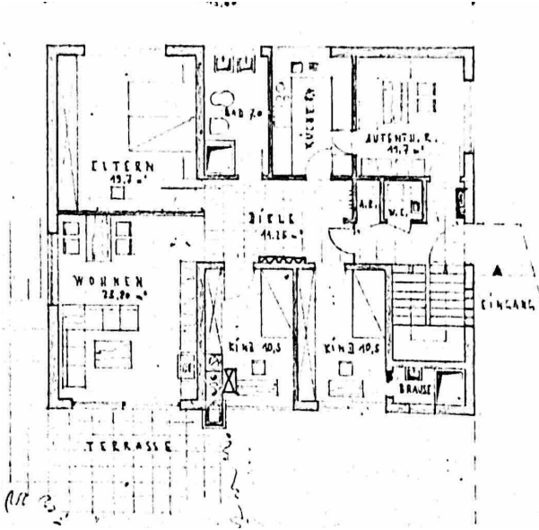
Erdgeschoss
