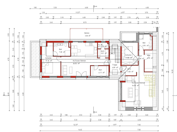
Grundriss Dachgeschoss
