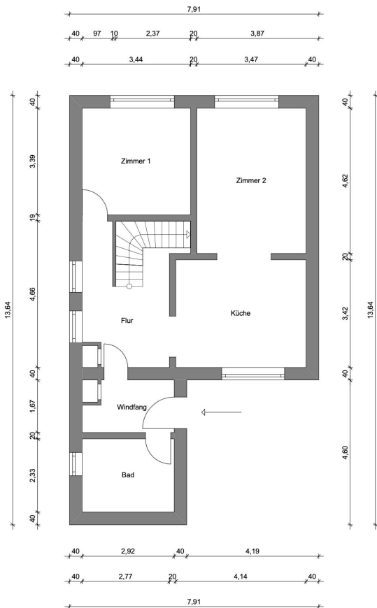
Grundriss Erdgeschoss
