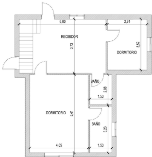
PLANTA BAJA ESCALAS 1/75 74.7 m 2
