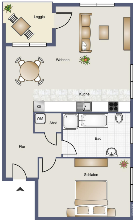
Grundrisskizze
