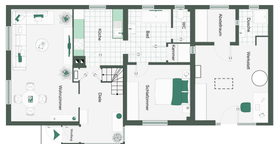
Erdgeschoss
