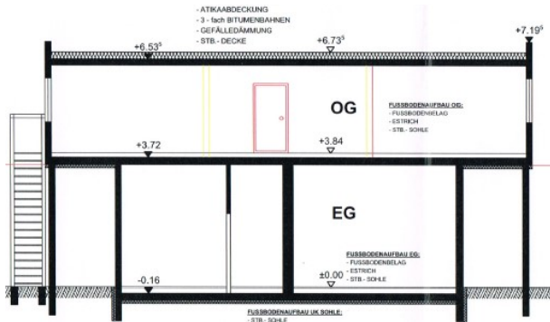
Schnitt
