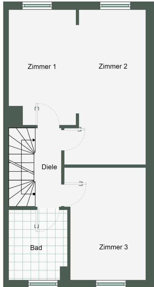
Grundriss OG
