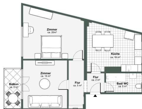
Grundriss
