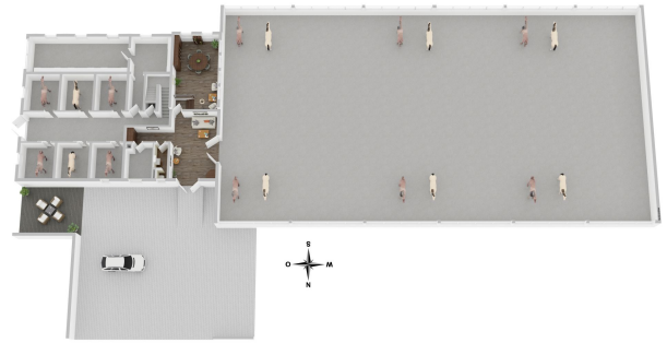
Grundriss Reithalle/Pferdeboxen
