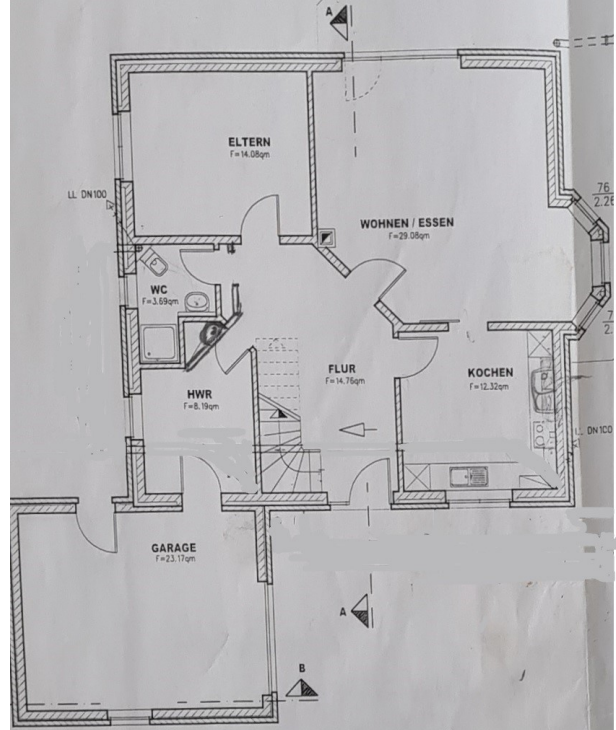
Grundriss_EG
