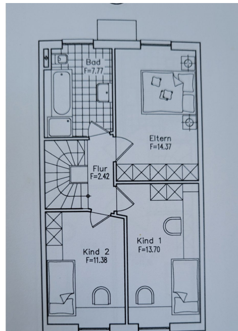
Grundriss_OG
