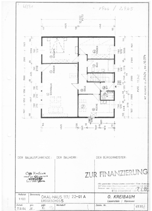
Grundriss_EG
