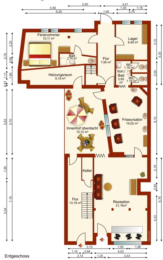
Grundriss Erdgeschoss
