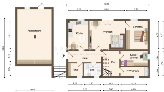
Grundriss Untergeschoss
