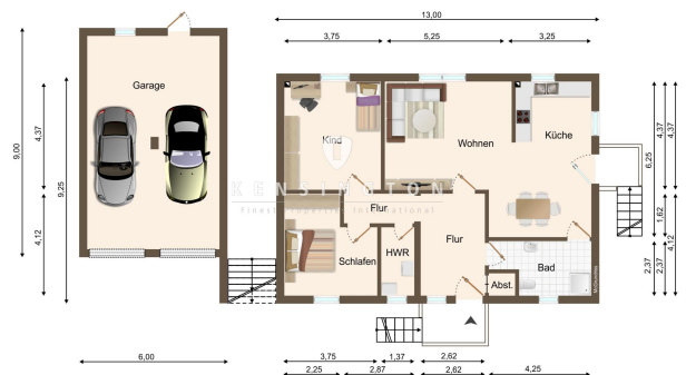
Grundriss Erdgeschoss
