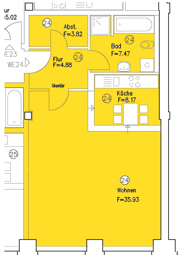
Grundriss
