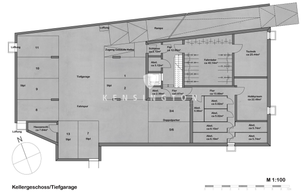
Untergeschoss / Tiefgarage
