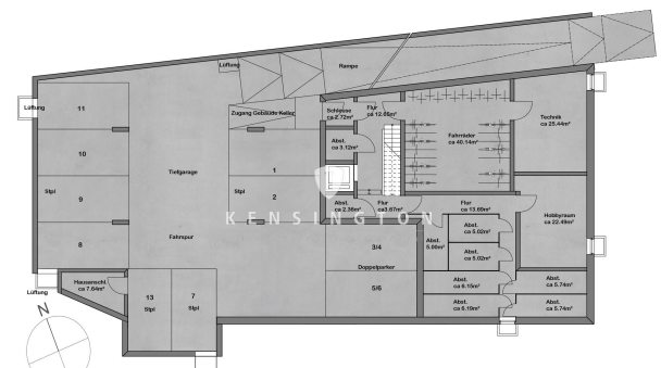
Kellergeschoss/Tiefgarage
