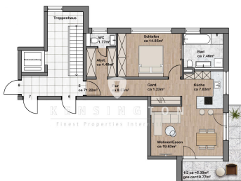
Wohnung Nr.5 Obergeschoss/ ca. 71.22m 2
