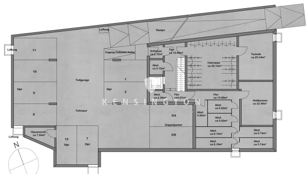
Kellergeschoss/Tiefgarage
