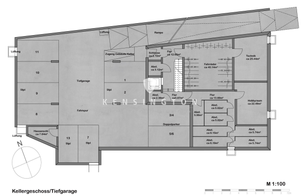
Untergeschoss / Tiefgarage
