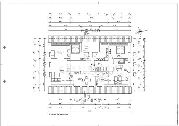
Obergeschoss
