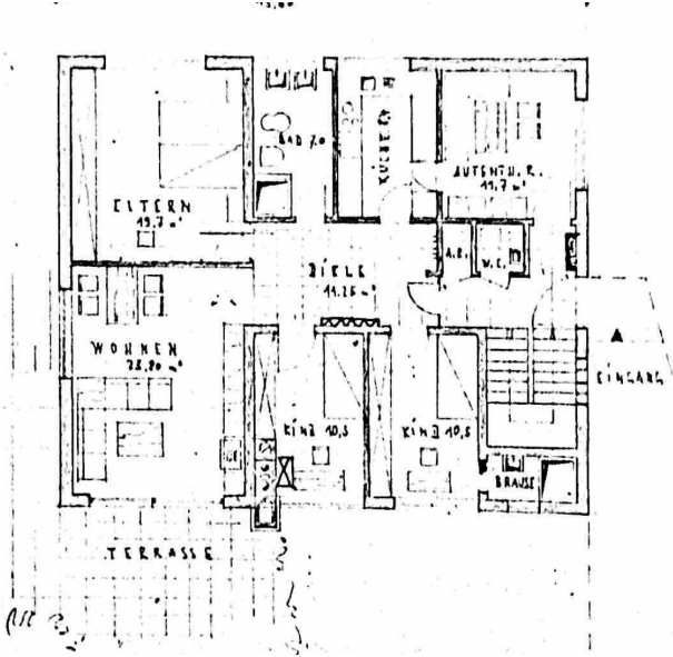
Erdgeschoss
