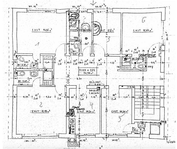
Obergeschoss
