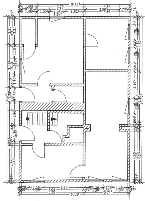
Grundriss Erdgeschoss
