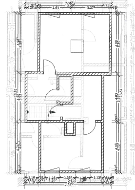
Grundriss Obergeschoss
