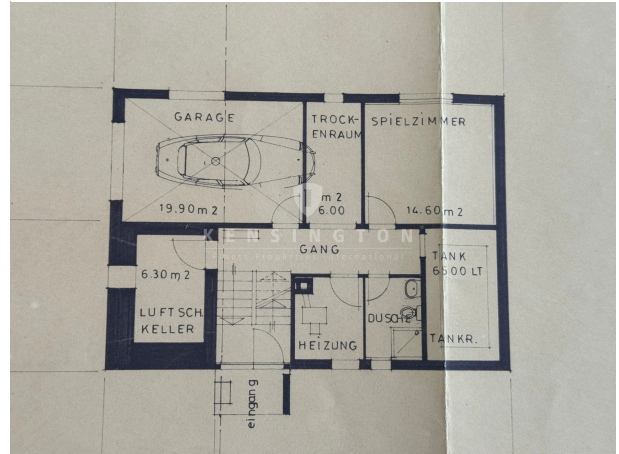
Grundriss UG
